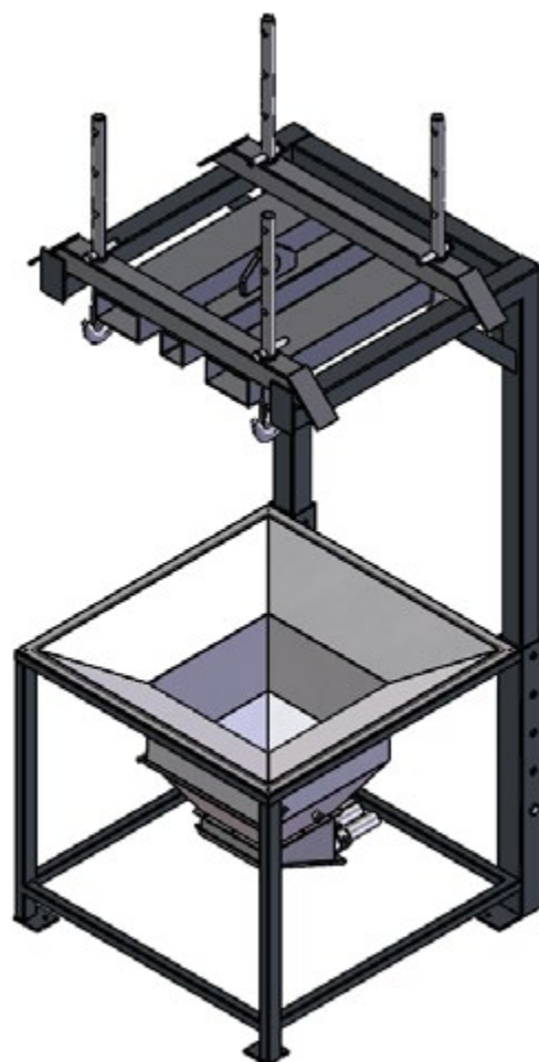
Die Entladestation ist höhenverstellbar
