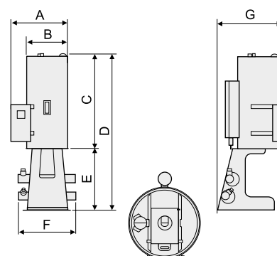
Deckel DH 200-800
