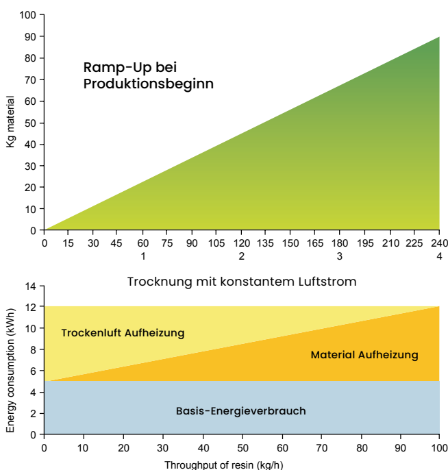
1: Standard Trockner mit konstanter Luftmenge.
