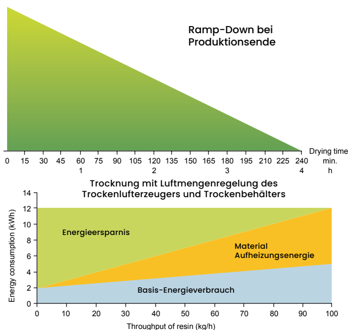
2: Trockner mit frequenzgeregeltem Gebläse, der die Luftmenge steuert.
