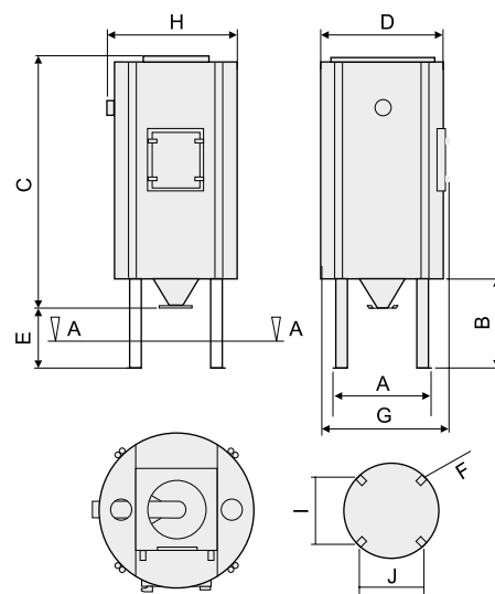
Deckel DH 1200-12000
